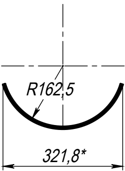
Поз.3 (Подушка)
