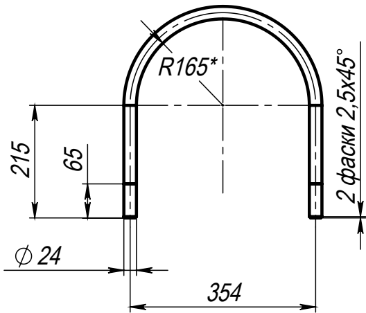
Поз.6 (Упор)
