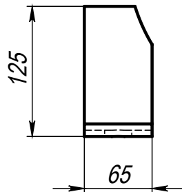
Поз.4 (Ушко) 1:5
